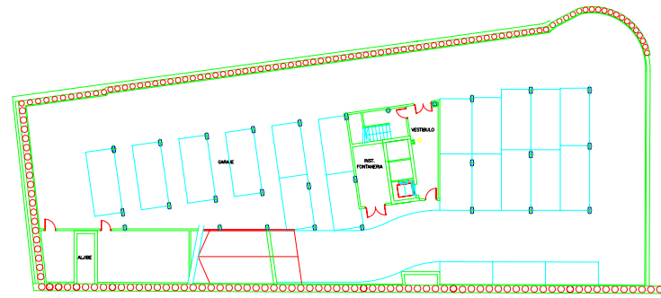
Planta Sotano
