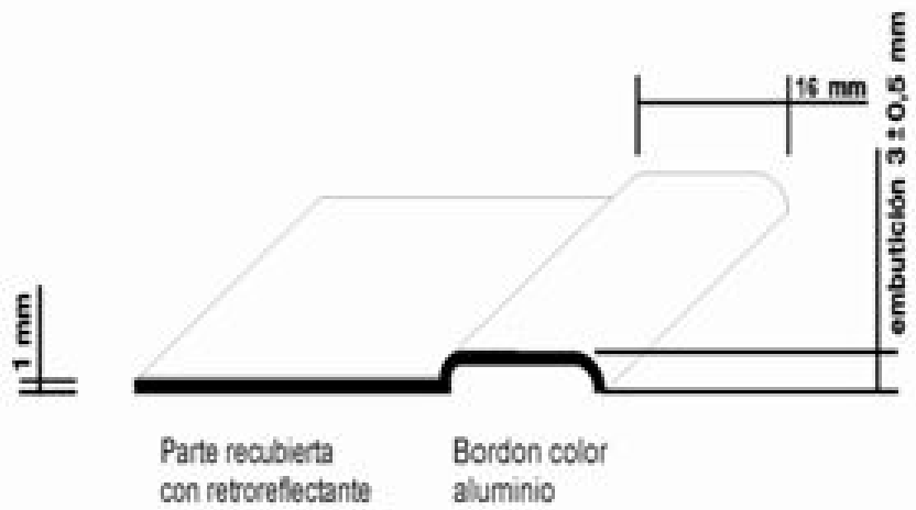
FIGURA 3 DETALLE BORDON PLACA
