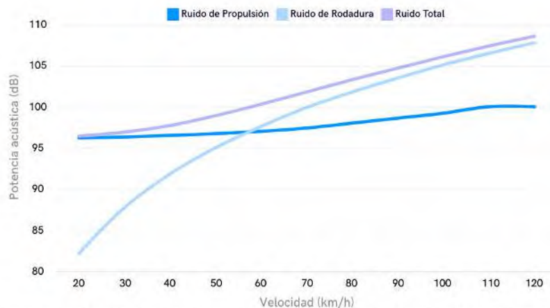
Figura 17. Relación entre el ruido de propulsión y rodadura con respecto a la velocidad para un vehículo categoría 1. Gráfica elaboración propia a partir de formulación de metodología CNOSSO-EU. 61
