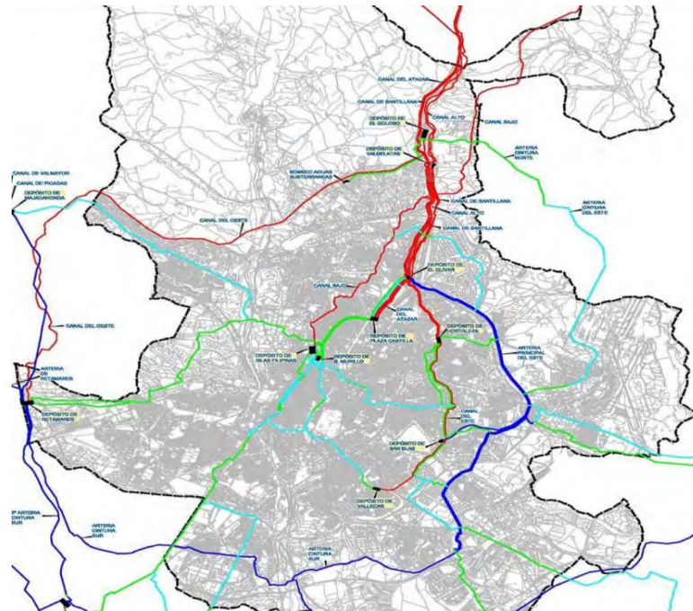
Figura 18 Esquema general arterias distribución
