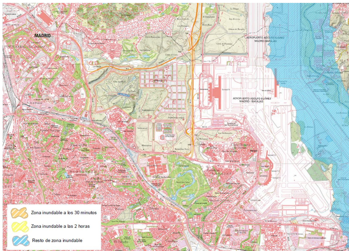
Figura 15 Delimitación de la Zona Inundable por la rotura de la Presa El Atazar
