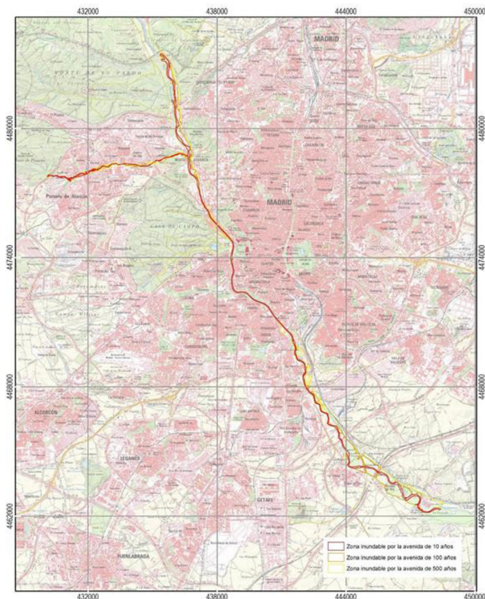
Figura 6 Delimitación de Zonas Inundables en el tramo ARPSI ES030-12-04.1-01
