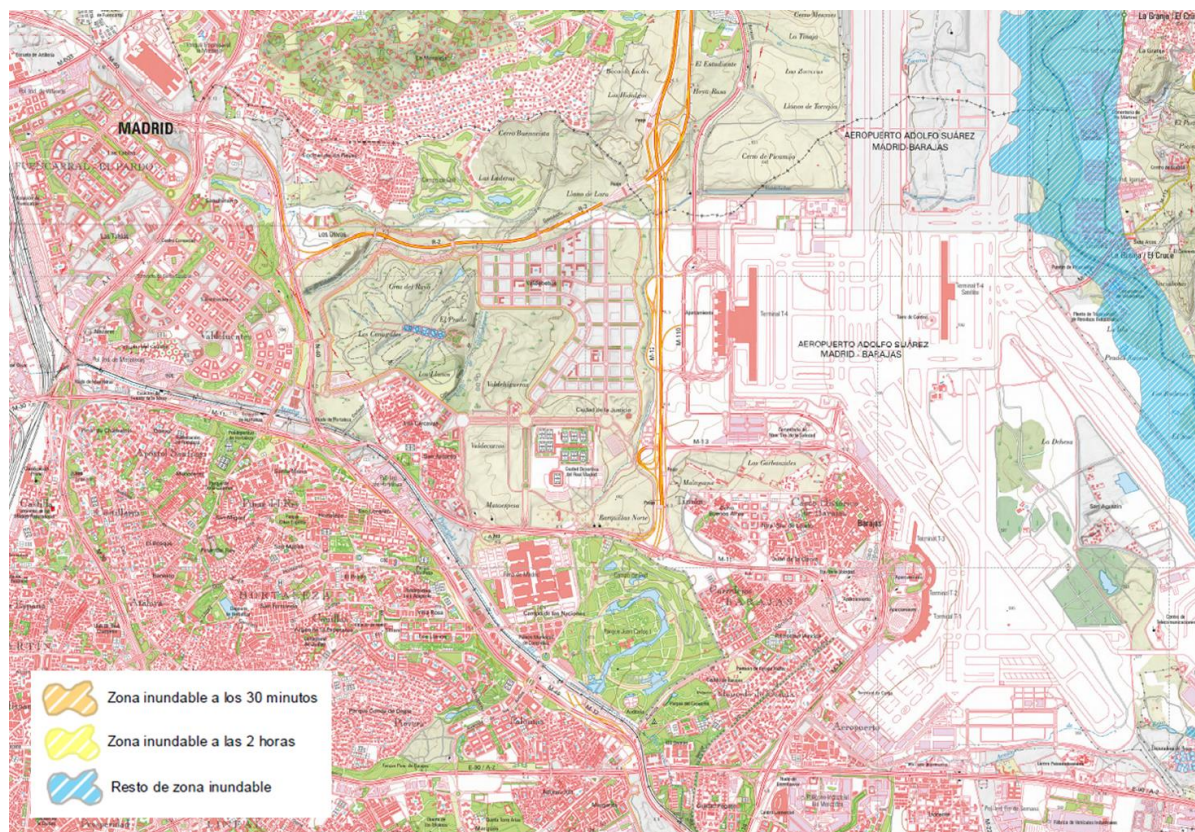
Figura 17 Delimitación de la Zona Inundable por la rotura del Embalse de Pedrezuela-El Vellón
