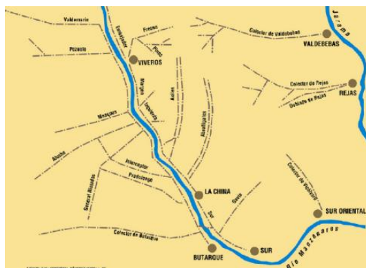
Figura 19 Esquema general colectores (FUENTE: Ayuntamiento de Madrid (Félix Cristóbal Sánchez))
