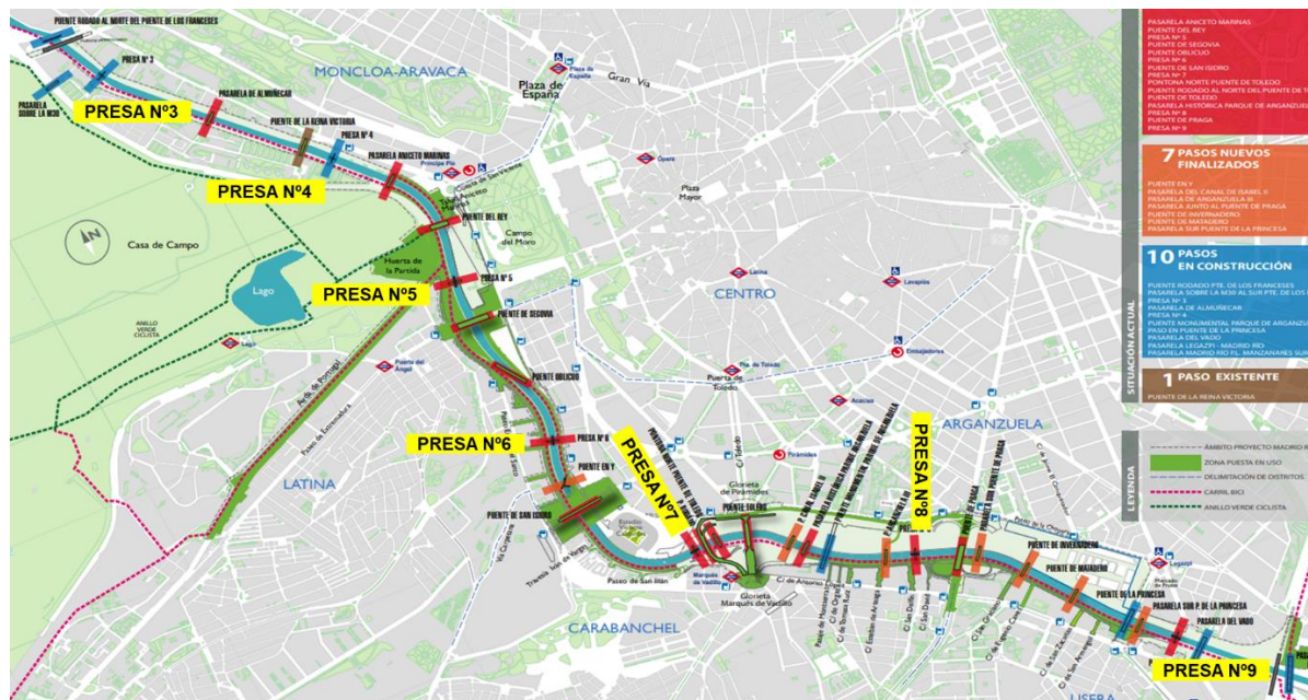
Figura 14. Ubicación Presas tramo urbano Madrid Río
