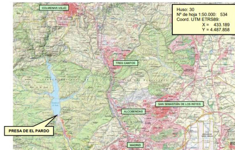
Figura 10. Situación de la Presa en el Mapa 1:50.000 del IGN
